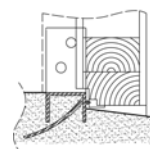
INGJUTET TRÖSKELJÄRN
