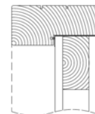
ÖVERSTYCKE
