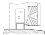
FRISTÄENDE TRÖSKELJÄRN
