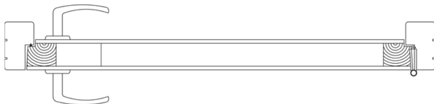
INGJUTET TRÖSKELJÄRN
