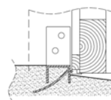
INGJUTET TRÖSKELJÄRN
